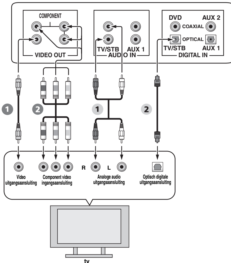
Achterpaneel van dit toestel
