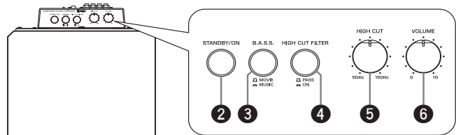
Bedienfeld
