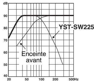
Graphique de réponse en fréquence*
