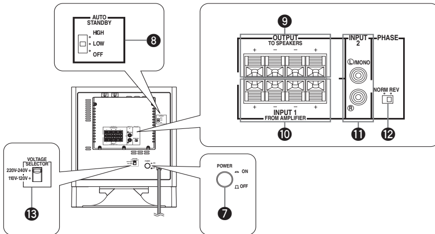
Panel trasero (Modelo básico)
