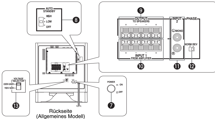
Bedienfeld
