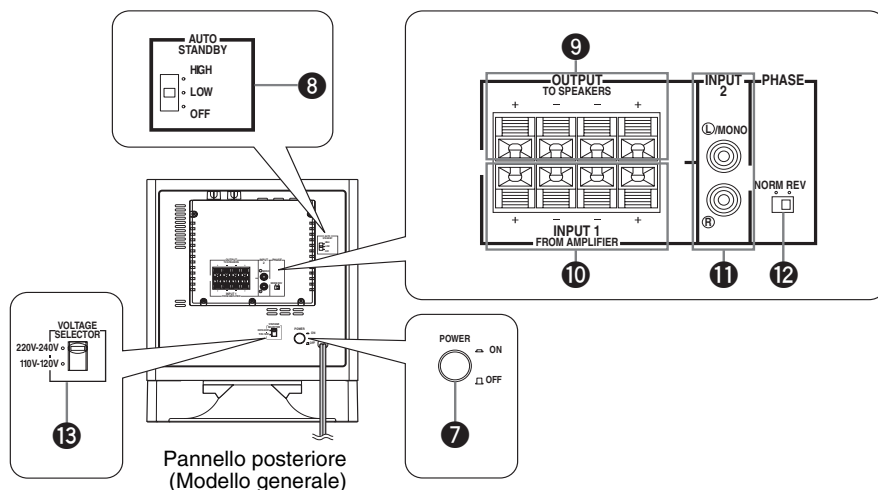
Pannello posteriore
