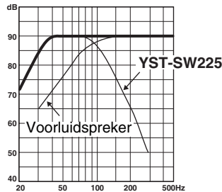
Diagram van de frequentiekaracteristieken*
