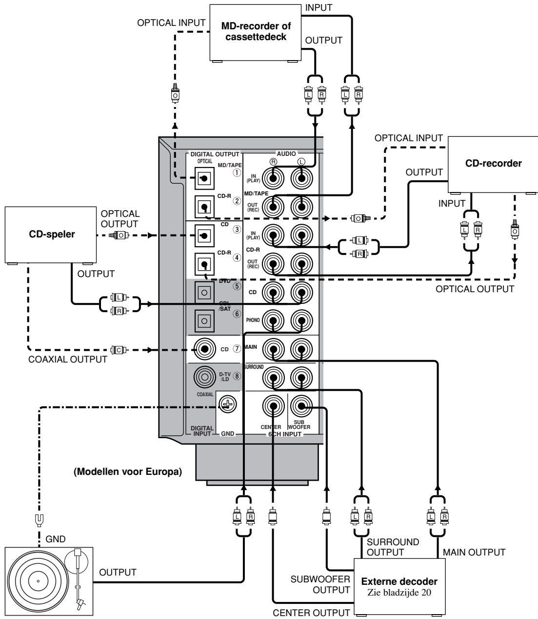
Draaitafel
