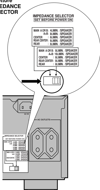
(Modello europeo)
